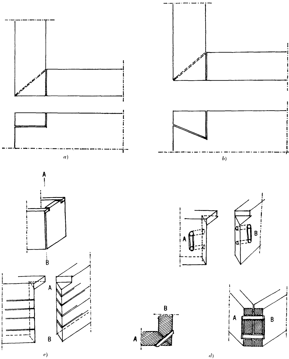
Fig. 9. -- Giunture agli angoli dei sarcofagi lignei. -- a, c ) Giunto ad angolo nascosto; b ) giunto ad angolo nascosto a coda di rondine; d ) giunto ad angolo nascosto con legature a buchi e scanalature rinforzate da cavicchi (LACAU, Sarcophages , I, p. 4, figg. 5,6)
