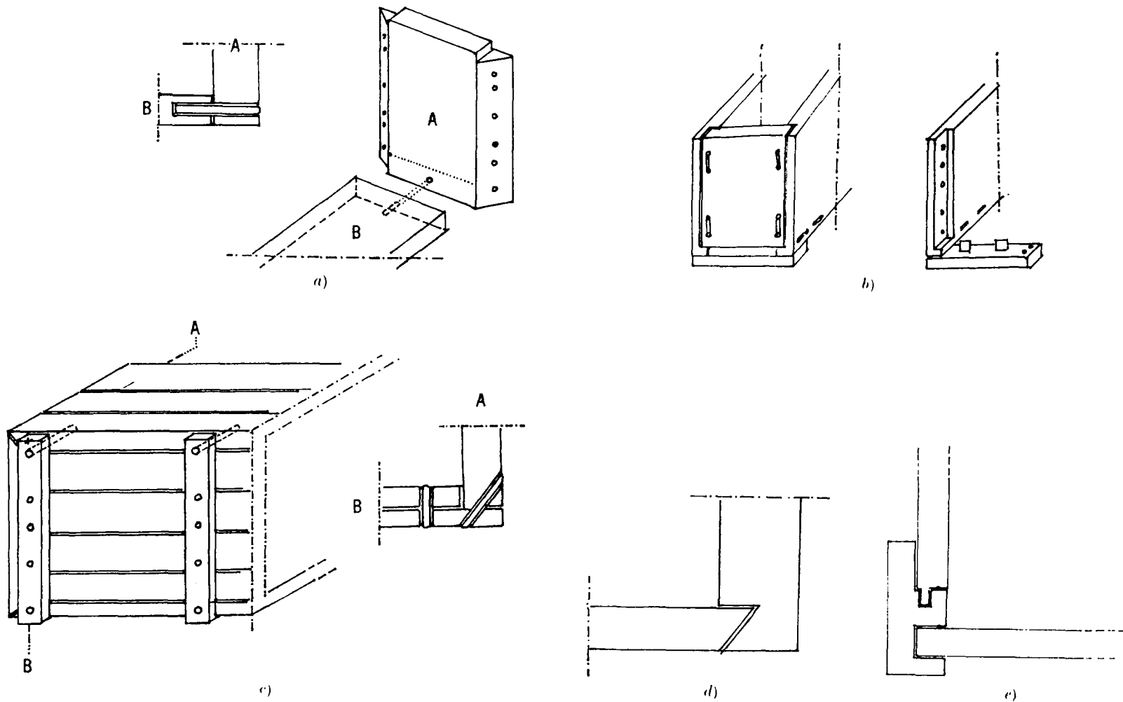
Fig. 10. – Metodi per unire fondo e lati dei sarcofagi lignei. – a) Giunto ad estremità diritte con cavicchi (LACAU, Sarcophages , I, p. 4, fig. 3); b) giunti a estremità diritte con lingue (LACAU, Sarcophages , II, p. 136, fig. 3); c) fondo e lati fissati con cavicchi ai tralicci di base (LACAU, Sarcophages , I, p. 4, fig. 4); d) incastro a mezza coda di rondine; e) fondo fissato in scanalature tagliate nello spessore delle pareti.
