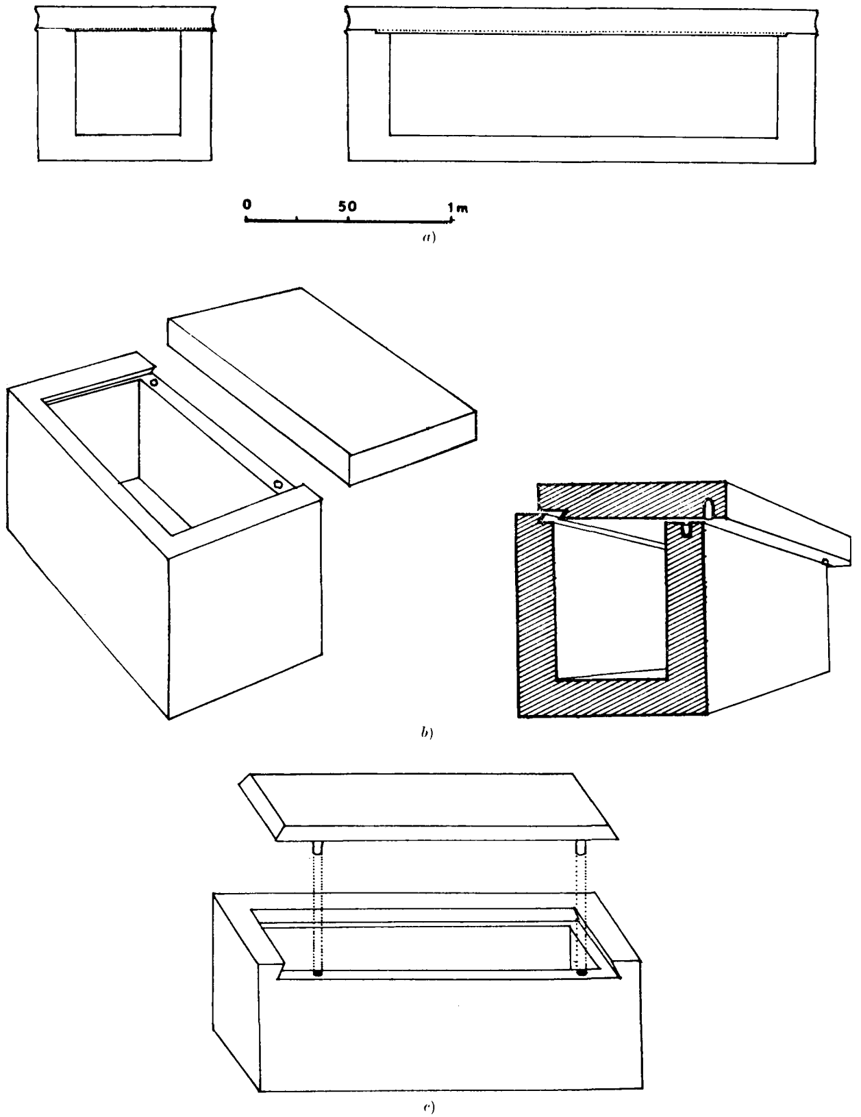
Fig. 13. - Chiusure di sarcofagi litici. - a) Sarcofago di Špšš-Pth (tipo C 3); b) sarcofago di Chefren (tipo C 4); c) Sarcofago anonimo (tipo C 5).
