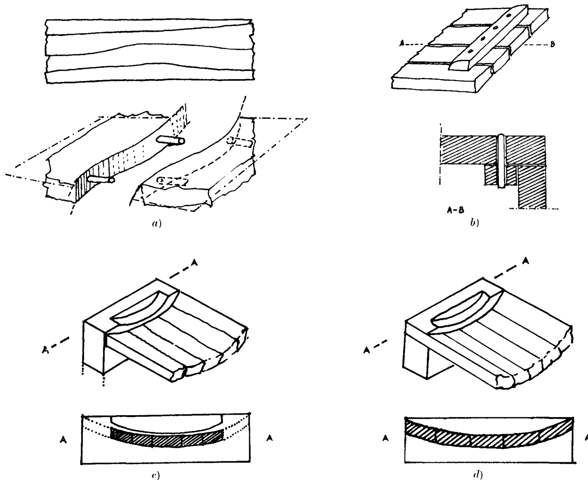
Fig. 11. - Coperchi. - a) Piano formato da assi unite con cavicchi (LACAU, Sarcophages , I, p. 3, fig. 1); b) piano con tasselli nella parte inferiore (LACAU, Sarcophages , I, p. 3, fig. 2); c) a volta, con assi incastrate parzialmente nello spessore delle pareti terminali; d) a volta, con assi incastrate nelle pareti terminali.
