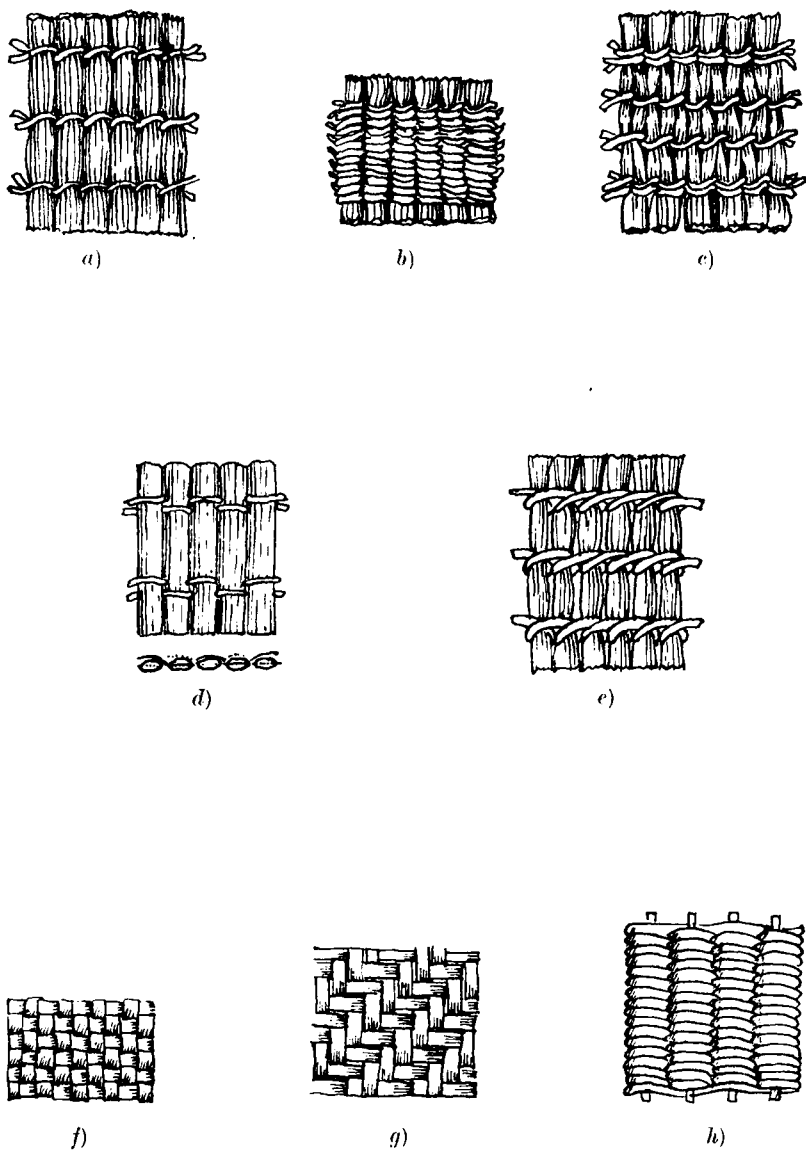
Fig. 1. - Tecniche di lavorazione delle stuoie. - Intrecciature incrociate: a) trama a fili distanziati; b) trama a fili ravvicinati; c) a mazzetti alternati; d) a canne forate. Intrecciatura ad avvolgimenti: e) a nodo rovescio. A «stuoia»: f) a scacchiera; g) a scala. A graticcio: h) con ordito rigido ( History of Technology , figg. 259-260).
