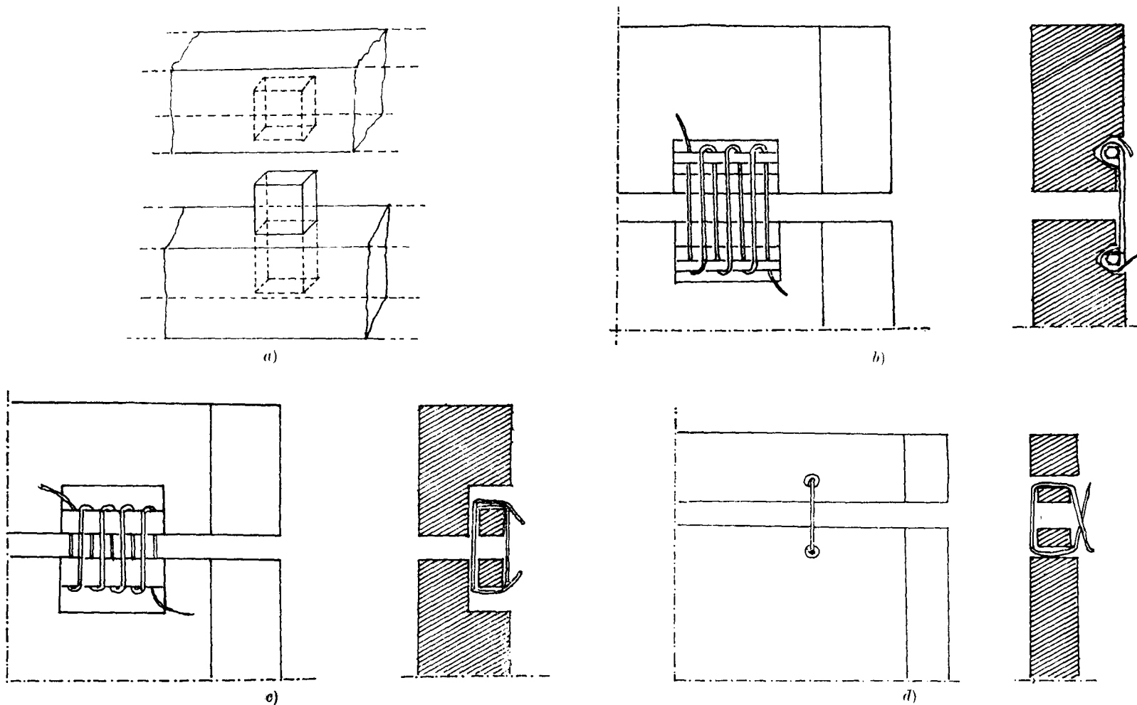
Fig. 7. — Metodi di unione delle tavole lignee formanti le pareti del sarcofago. — a) Con lingue piatte; b) cucitura a mortasa; c) cucitura a mortasa nascosta; d) cucitura a buchi e scanalature (PETRIE-MACKAY, Heliopolis , tav. XXV).
