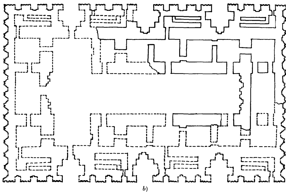
Fig. 18. - Piante di edifici a nicchie. - a) Egitto, Saqqāra, mastaba 3503 (EMERY, Great Tombs , II, tav. XXXVIII); b) Mesopotamia, Uruk, E-Anna, tempio D (E. HEINRICH, Zeitschrift für Assyriologie , n. s. XV, 1950, tav. 2).
