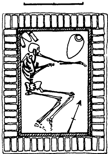
Fig. 6. – Passaggio dal rivestimento ligneo della camera funeraria al sarcofago. – a) Camera funeraria con rivestimento ligneo. Šaqqāra, tomba sussidiaria 3506-1; b) camera funeraria con sarcofago ligneo. Šaqqāra, tomba sussidiaria 3506-5 (EMERY, Great Tombs , III, tavv. 45, 49).
