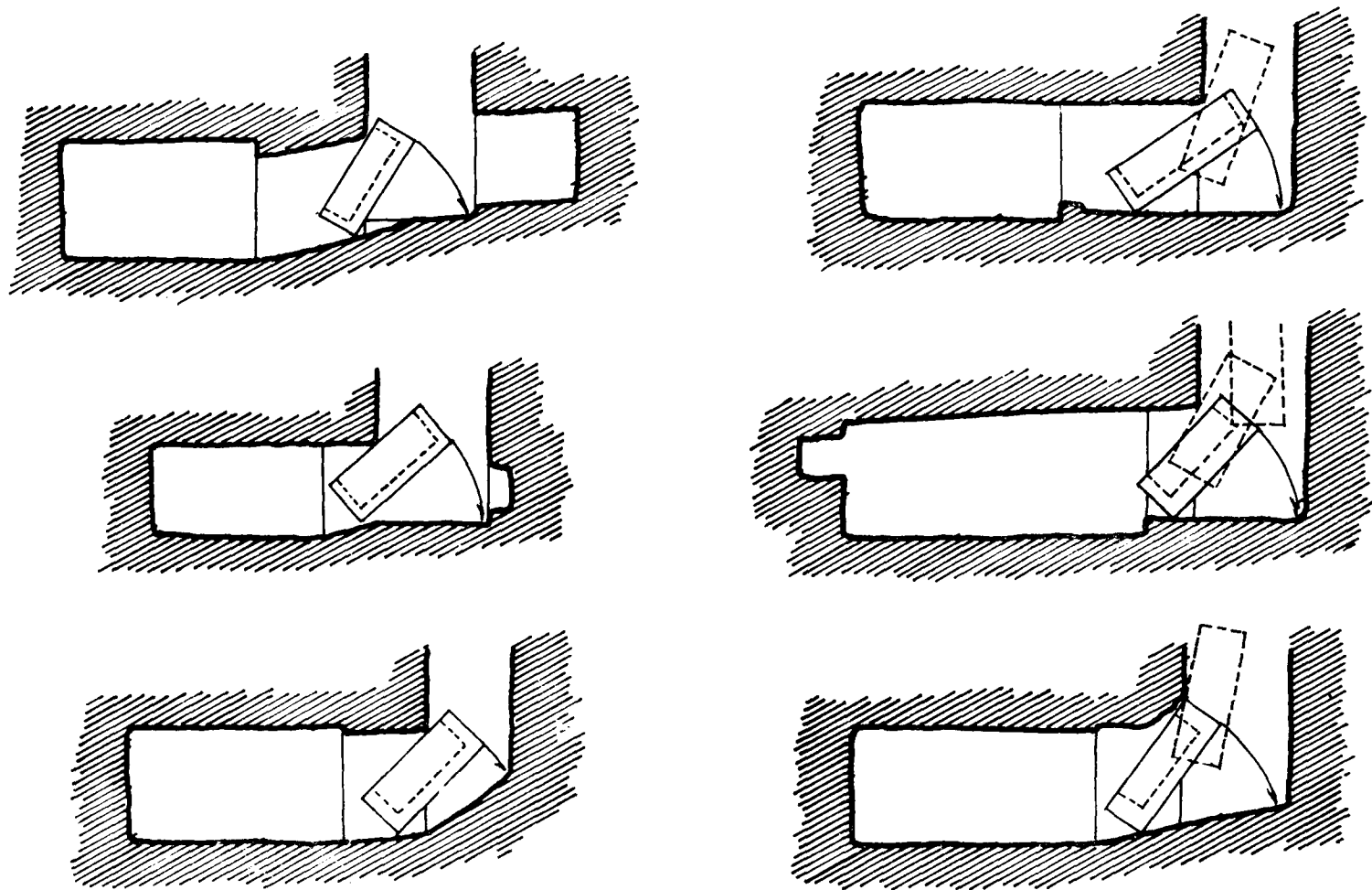
Fig. 16. - Metodi per far scendere il sarcofago lungo il pozzo fino alla camera funeraria (JUNKER, Giza , X, fig. 14).
