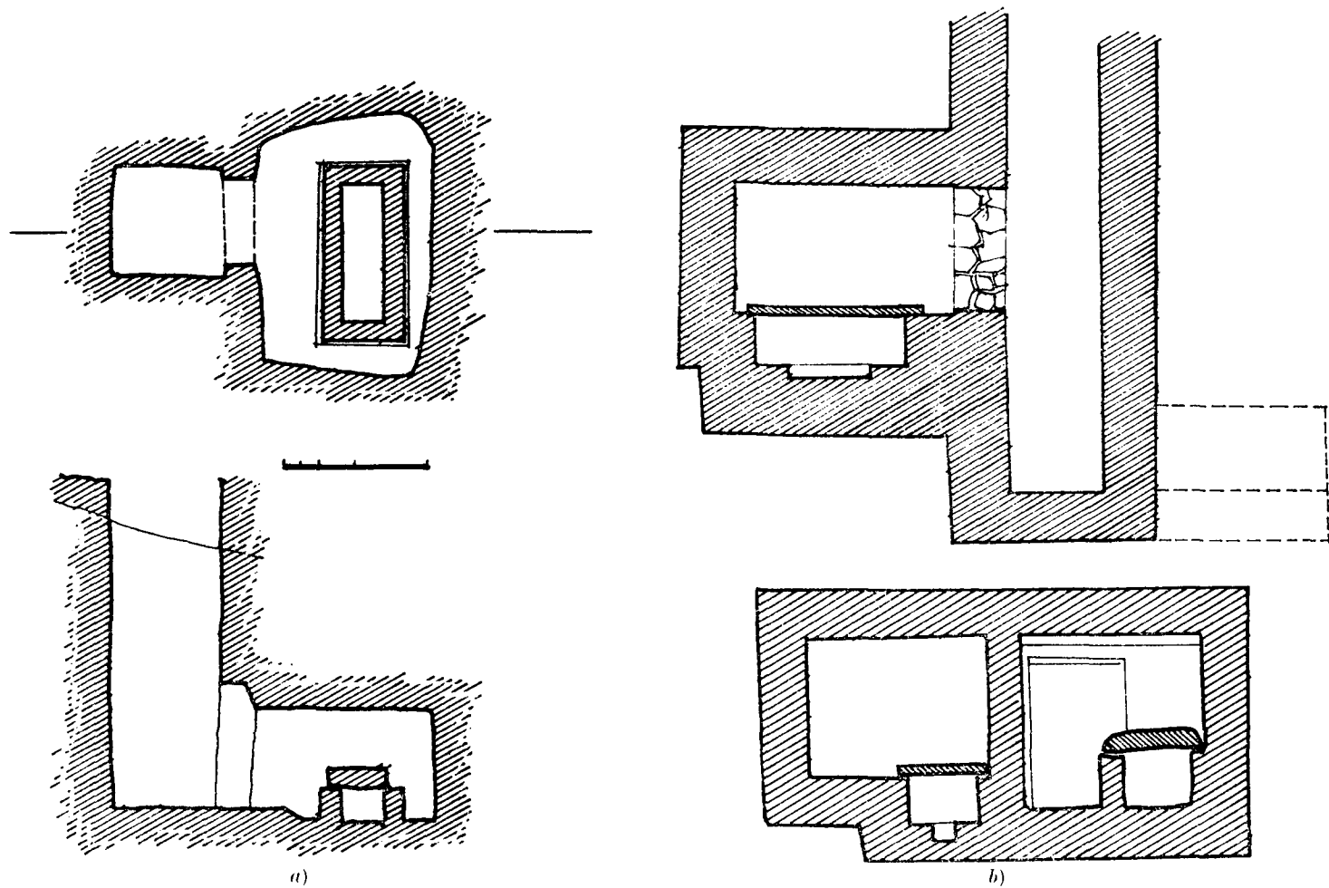
Fig. 15. - Sarcofagi ricavati nella roccia viva della camera funeraria. - a ) Risparmiato nello scavo della camera (JUNKER, Giza , VIII, fig. 24); b ) tagliato nel pavimento (JUNKER, Giza , VI, fig. 65).
