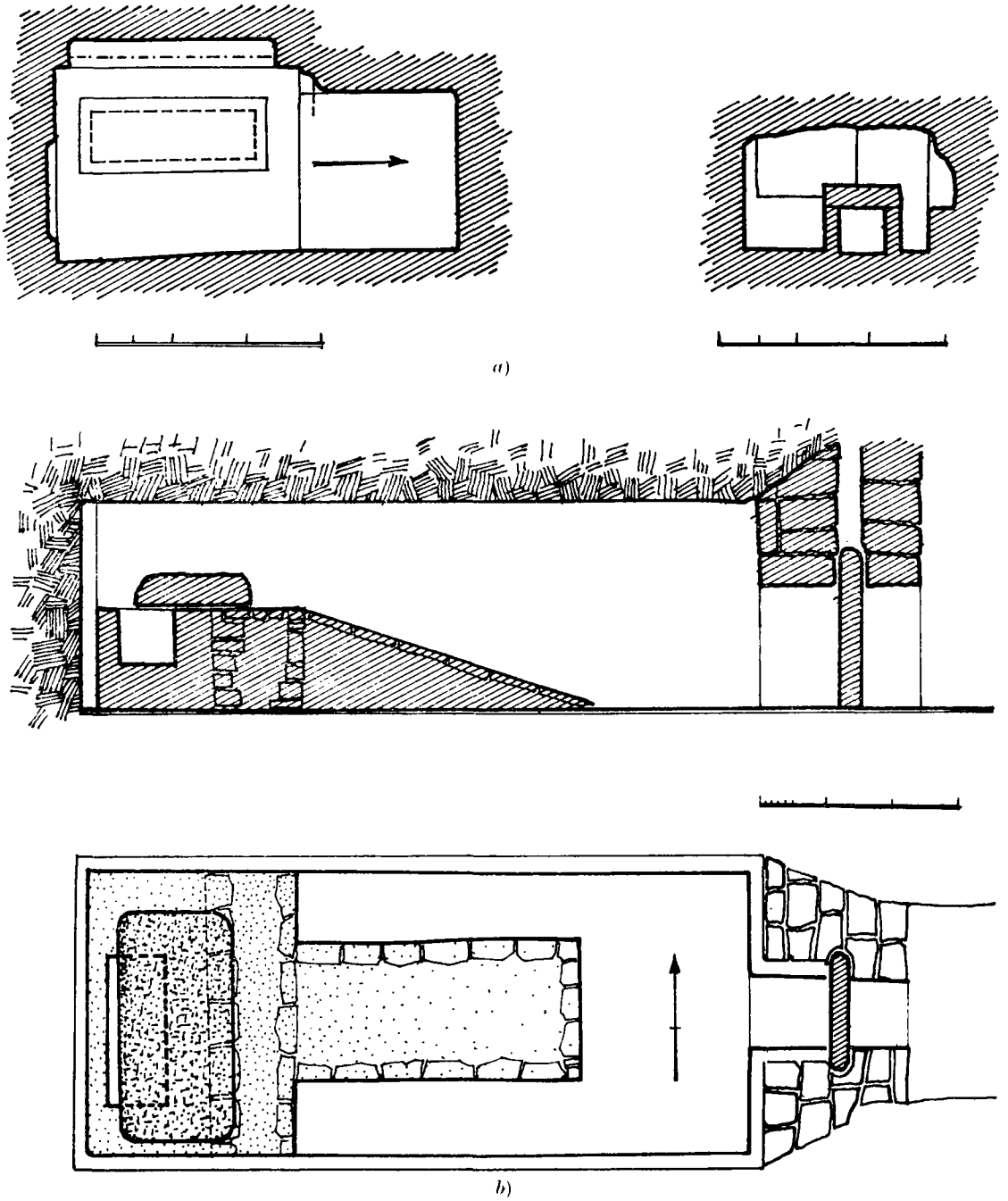
Fig. 17. - Metodi per collocare il coperchio sui sarcofagi litici. - a) Nicchia nella parete ovest della camera funeraria (JUNKER, Giza , VII, fig. 77); b) con uno scivolo davanti alla parete est del sarcofago (FIRTH-GUNN, Teti Pyramid Cemeteries , fig. 19).
