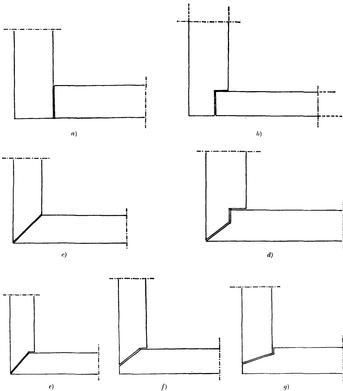
Fig. 8. - Giunture agli angoli dei sarcofagi lignei. - a) Giunto a estremità diritte; b) giunto a mezzo legno; c) giunto ad angolo o a quartabono; d) giunto ad angolo con doppia spalla; e-g) giunti ad angolo con spalla (PETRIE-MACKAY, Heliopolis , tav. XXV).
